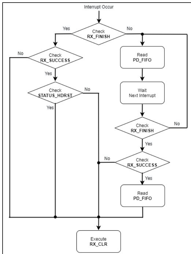
图. 5.14: RX 流程图
