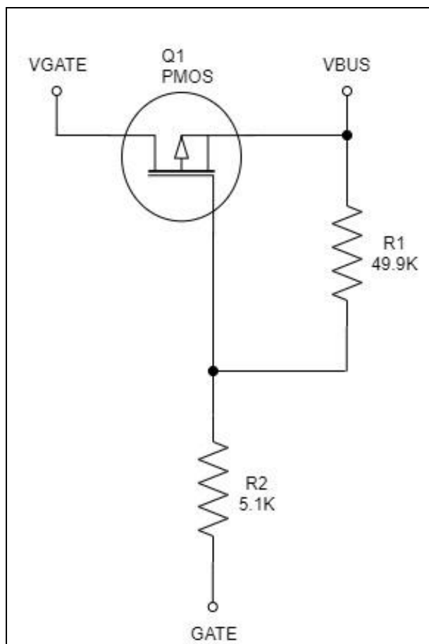
图 5.17: GATE 引脚应用连接示意图
