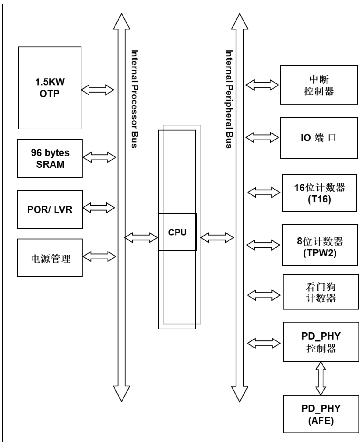
图. 2.1: PUD310 架构图
